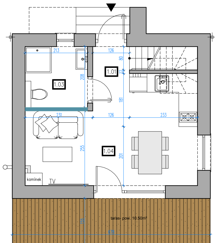
RZUT PARTERU
